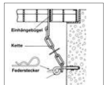
Sicherungsketten verzinkt, schnell und ohne Werkzeug lösbar. Bestehend aus: Flacheisenhaken mit Kette, Ösenschaube und Dübel; Gesamtlänge ca. 80cm; paarweise verpackt mit Montageanleitung
